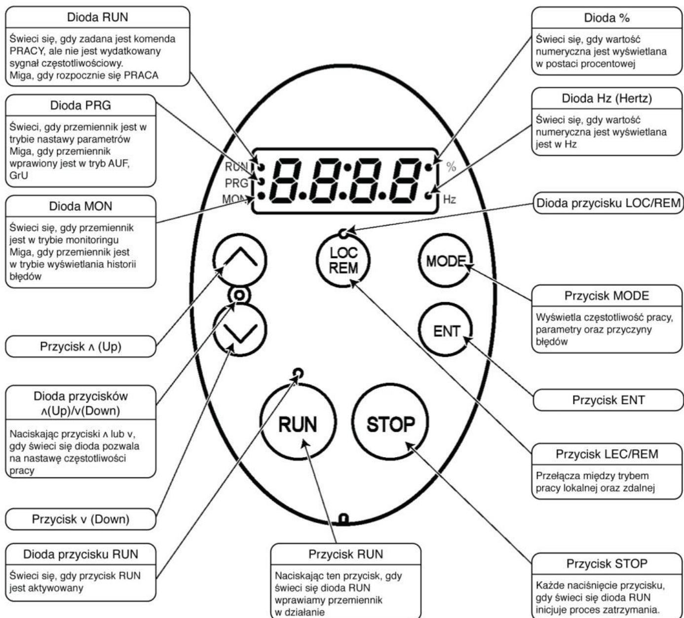
Rys. 9 Opis panelu sterującego przemiennika częstotliwości
