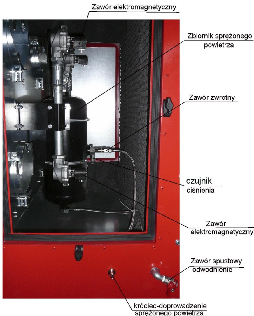
Rys. 3 Instalacja pneumatyczna
