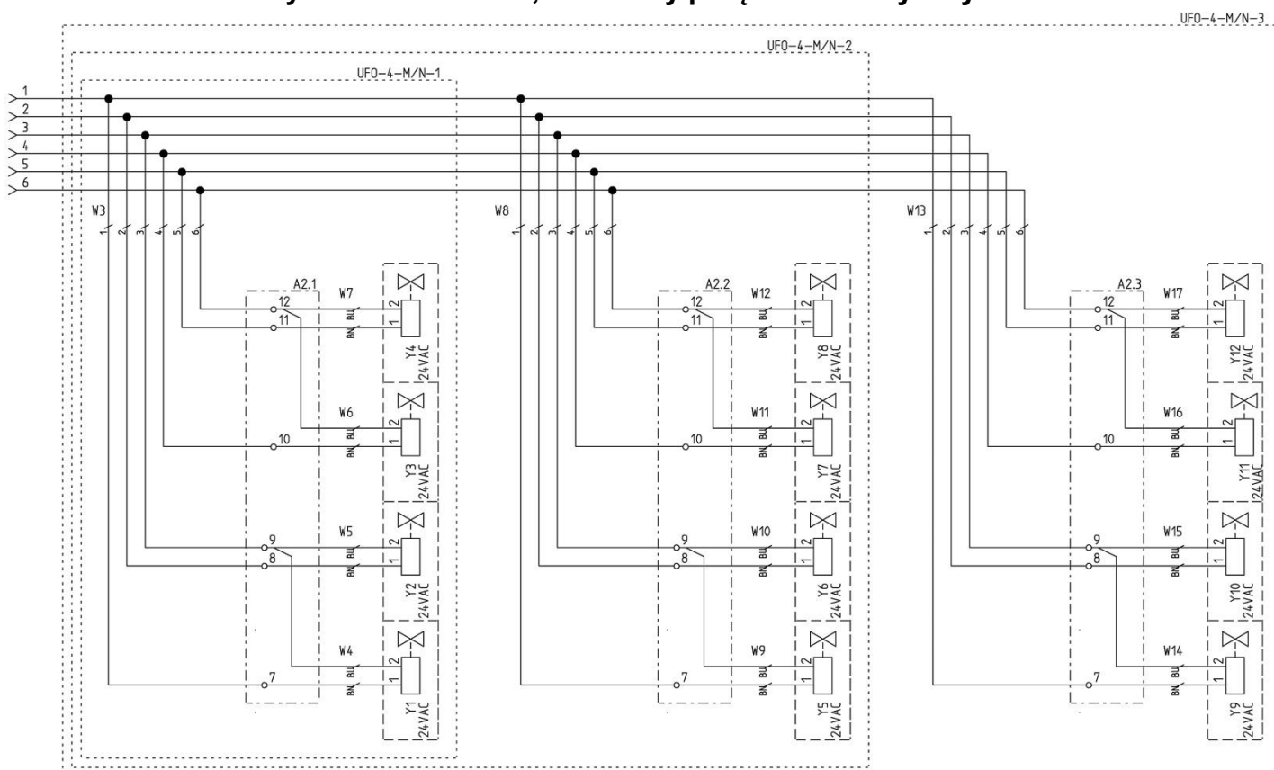
Rys. 5 UFO-4-M/N-3, Podłączenie elektrozaworów
