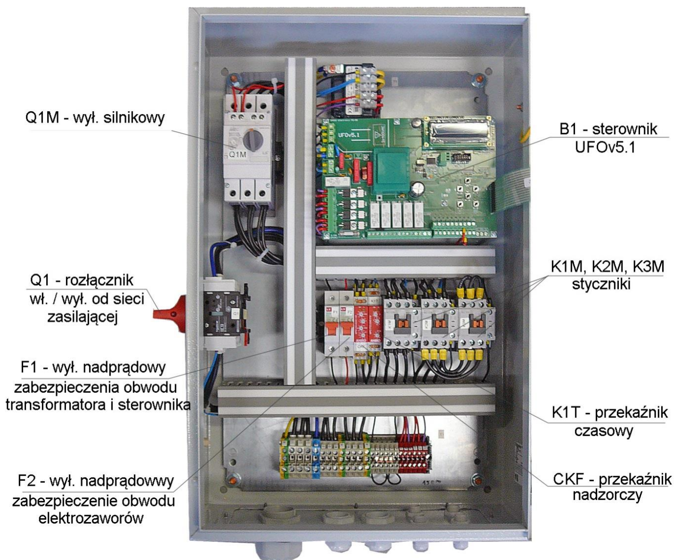
Rys. 8 Zespół elektryczny ZE-UFO-4-M/N-3, wewnątrz
