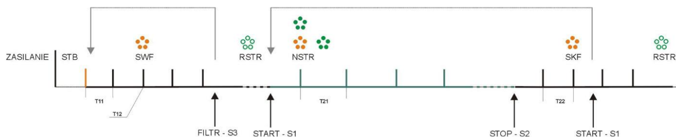
Rys. 9 Przebieg czasowy stanów prac
