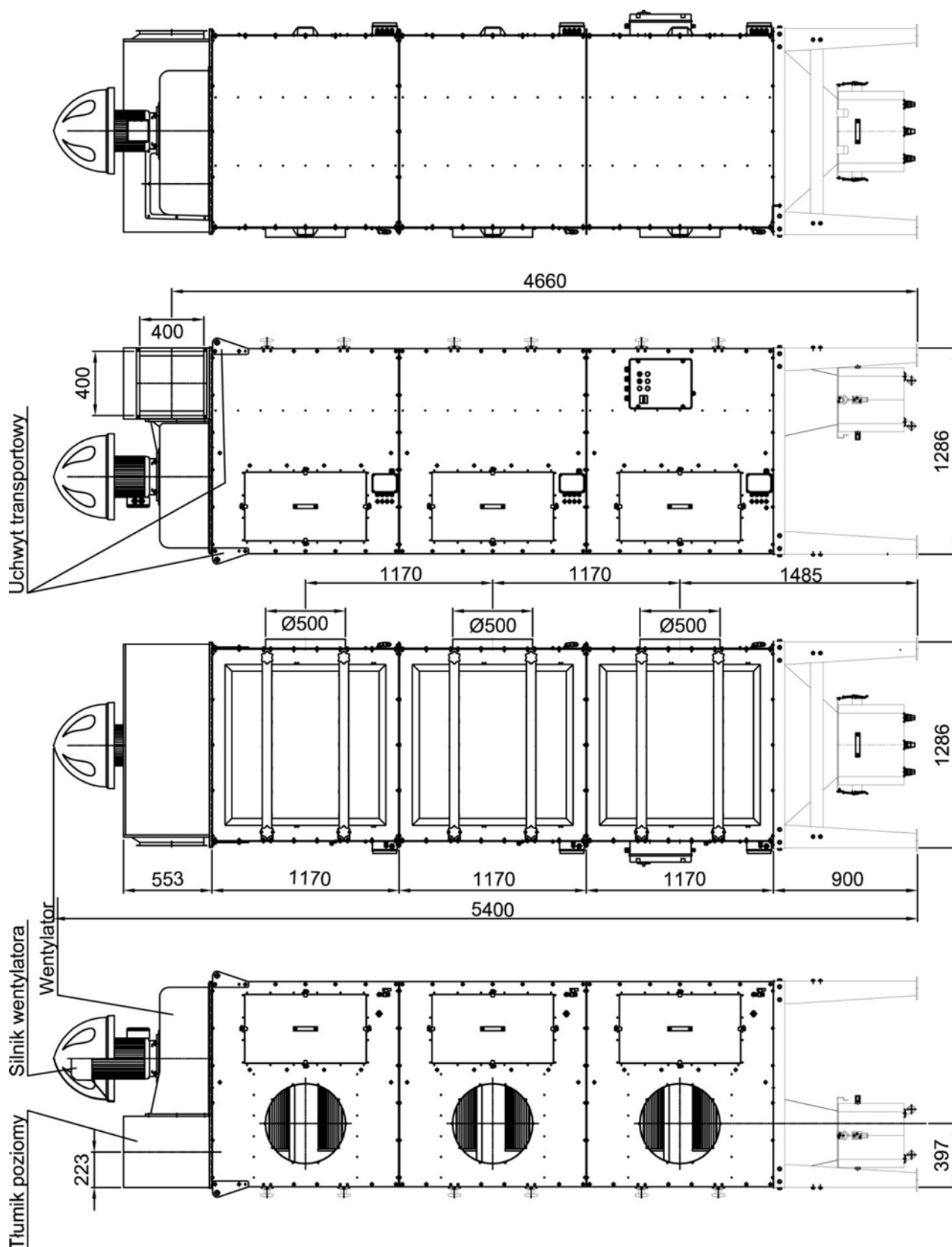
Rys. 1. UFO-4-M/N-3, budowa i wymiary
