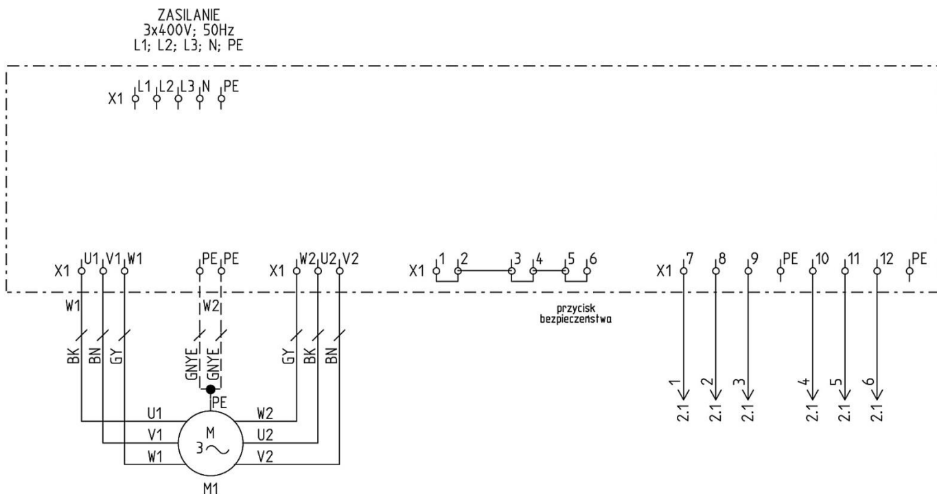
Rys. 4 UFO-4-M/N-3, schematy połączeń elektrycznych
