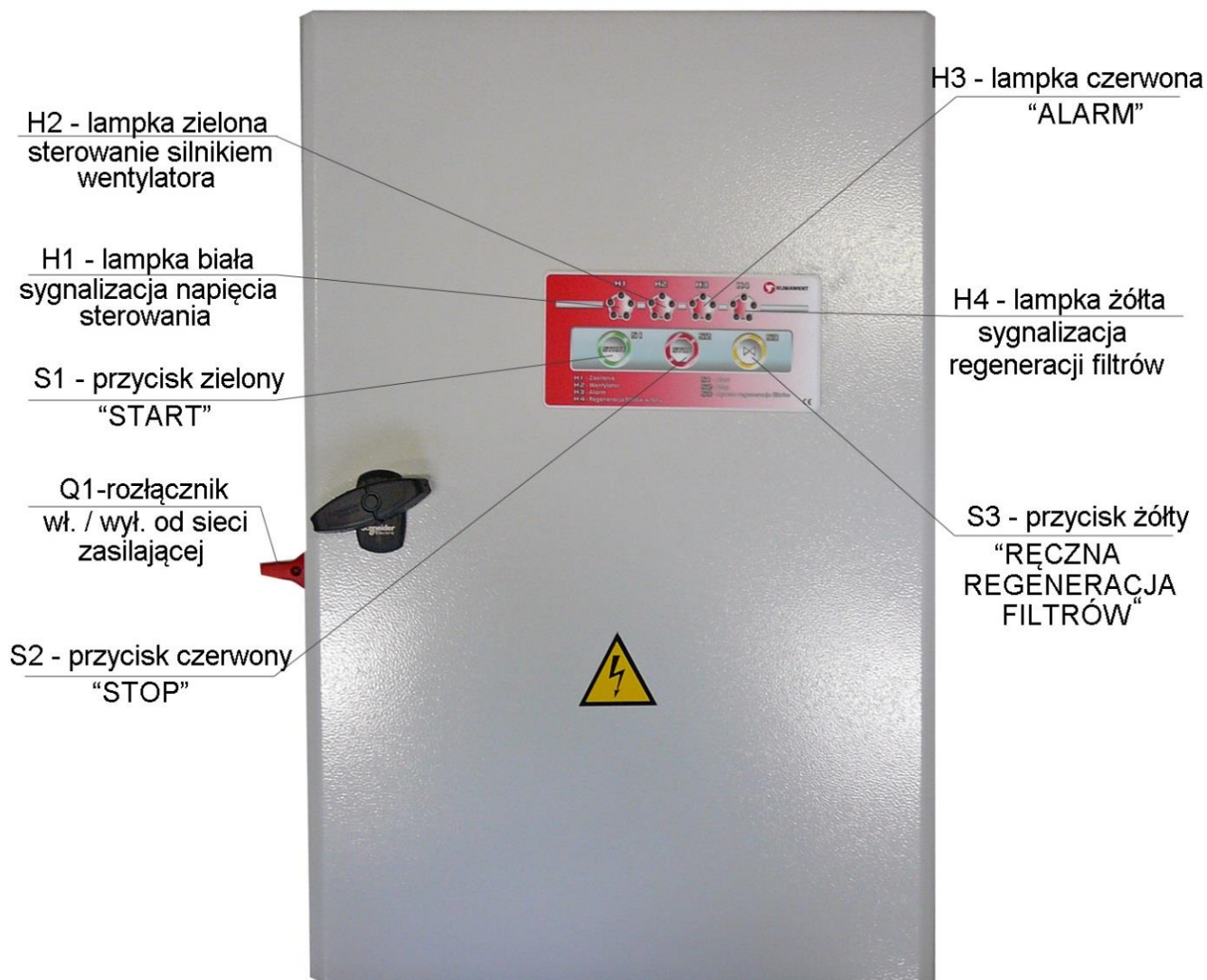
Rys. 6 Zespół elektryczny ZE-UFO-4-M/N-3, elewacja
