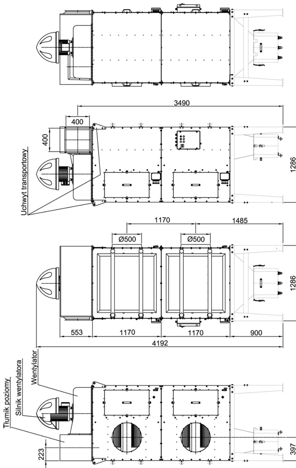
Rys. 1. UFO-4-M/N-2/R, budowa i wymiary
