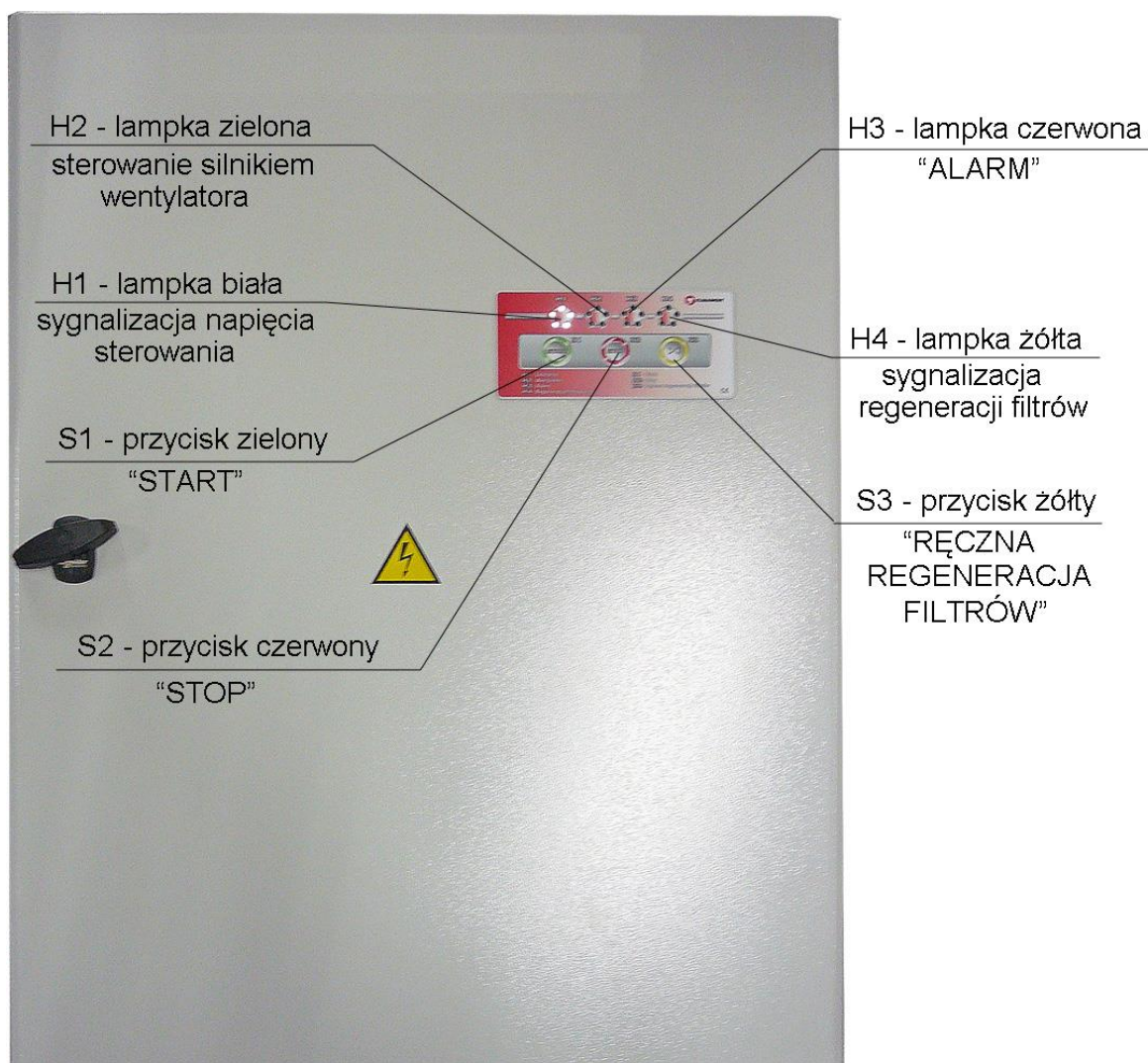
Rys. 6 Zespół elektryczny ZE-UFO-4-MN-2/R, elewacja
