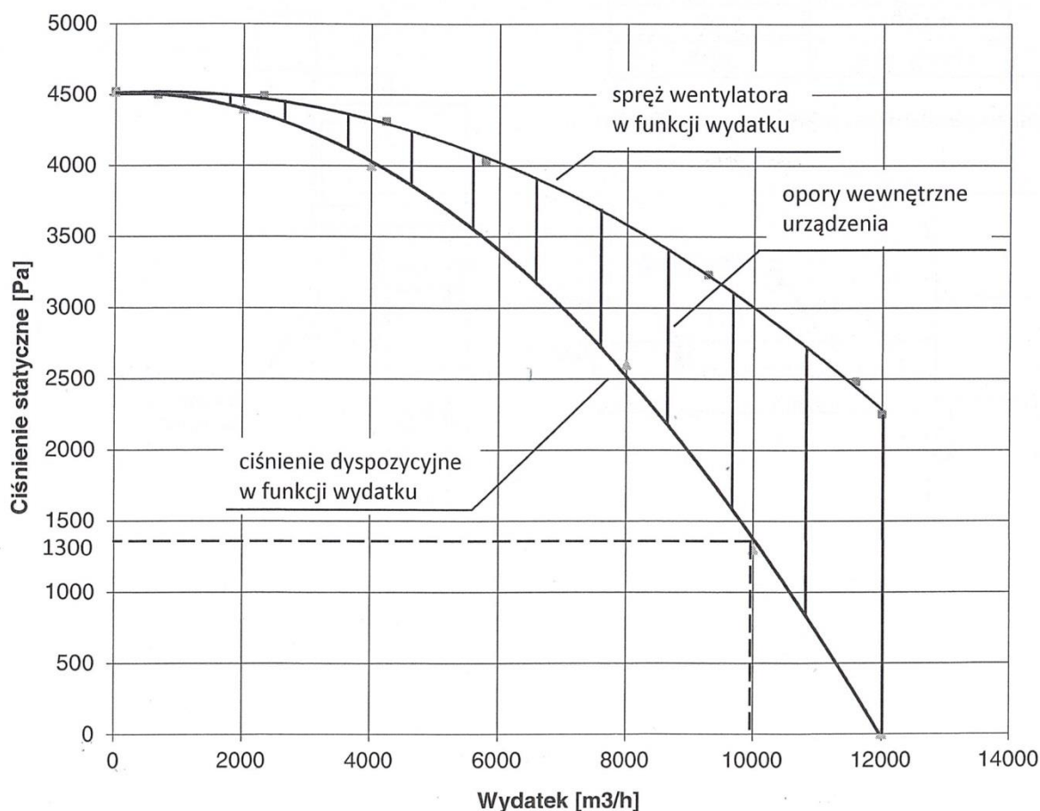
Charakterystyka przepływowa
