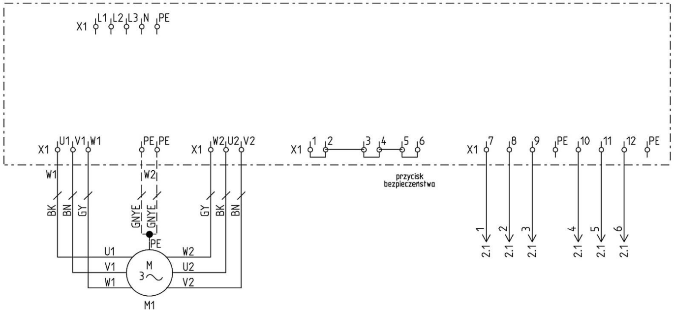
Rys. 4 UFO-4-M/N-2, schemat połączeń elektrycznych
