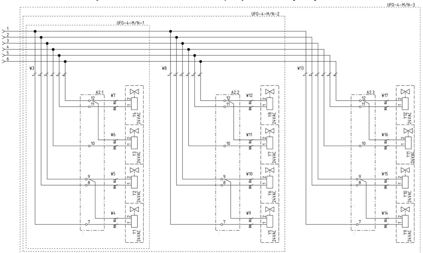
Rys. 5 UFO-4-M/N-2, Podłączenie elektrozaworów
