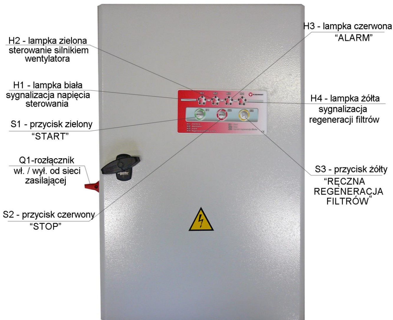
Rys. 6 Zespół elektryczny ZE-UFO-4-MN-2, elewacja
