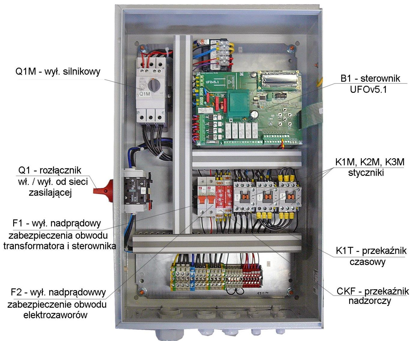
Rys. 8 Zespół elektryczny ZE-UFO-4-M/N-2, wewnątrz
