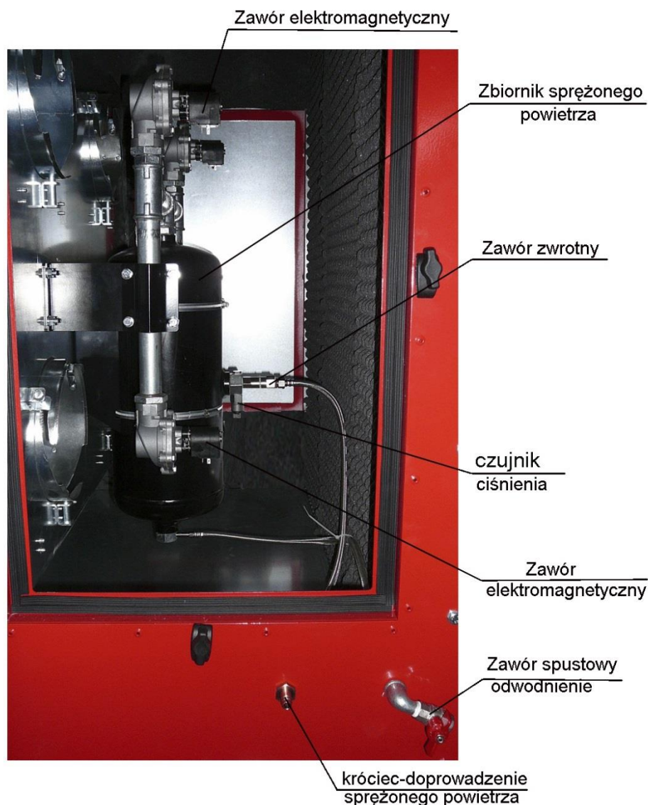
Rys. 3 Instalacja pneumatyczna
