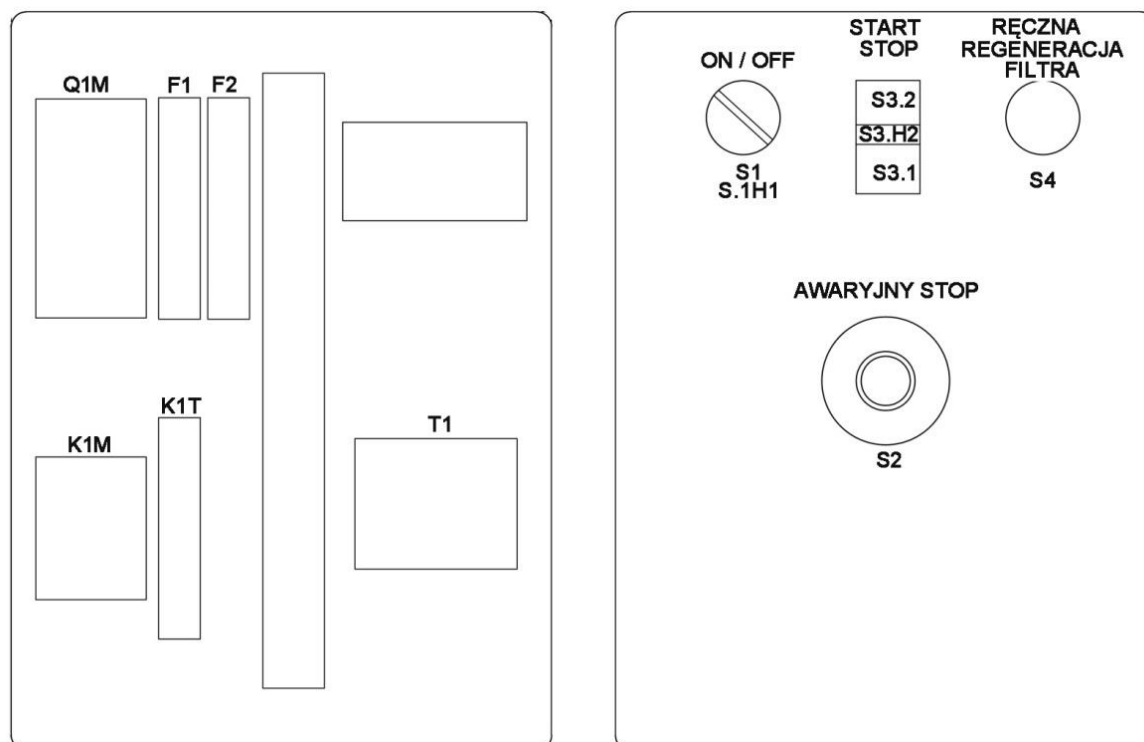
Rys.5 ZE-UFO-1-MN-HN-S, Zabudowa aparatury
