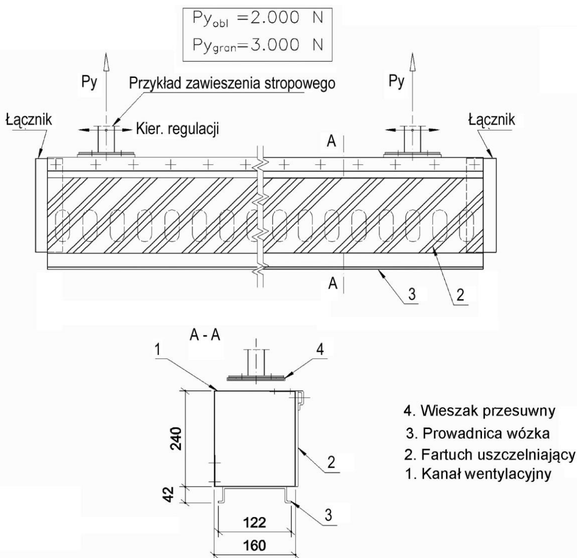
Rys.1 Kanał odciągowy samouszczelniający KOS-L
