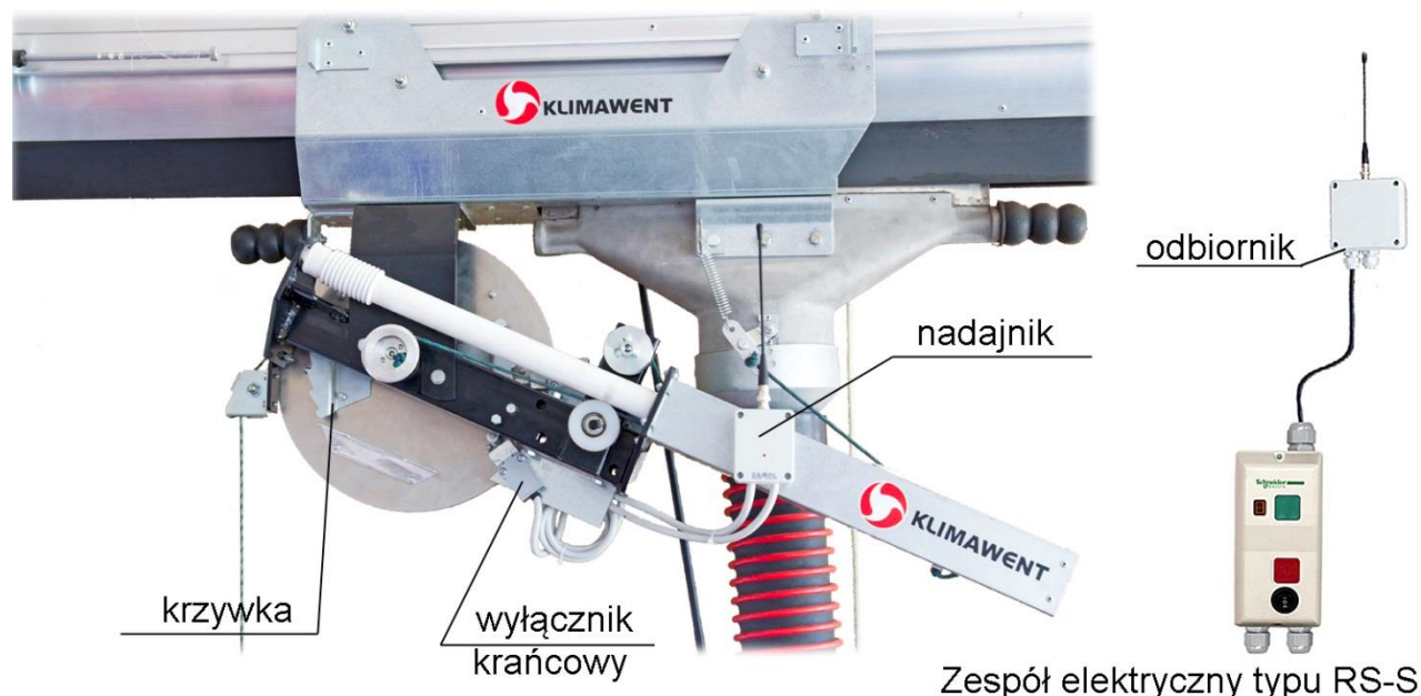
Rys. 2 Sterowanie radiowe pracą wentylatora
