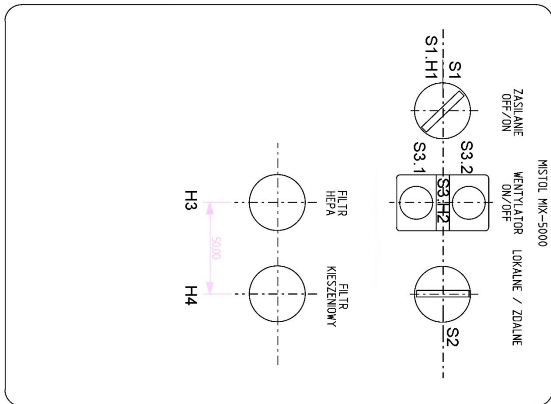
Rys. 4 Zespół elektryczny urządzenia typu MISTOL MIX-5000
