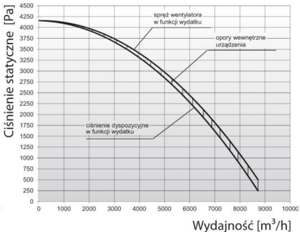
Rys. 1 Charakterystyka przepływowa urządzenia typu MISTOL MIX-5000
