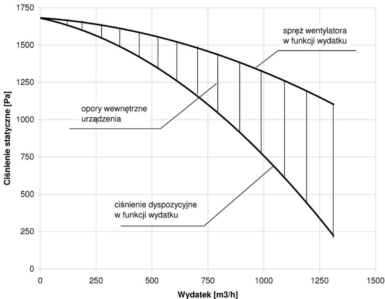
Rys. 1 Charakterystyka przepływowa urządzenia typu HARD-1000-S
