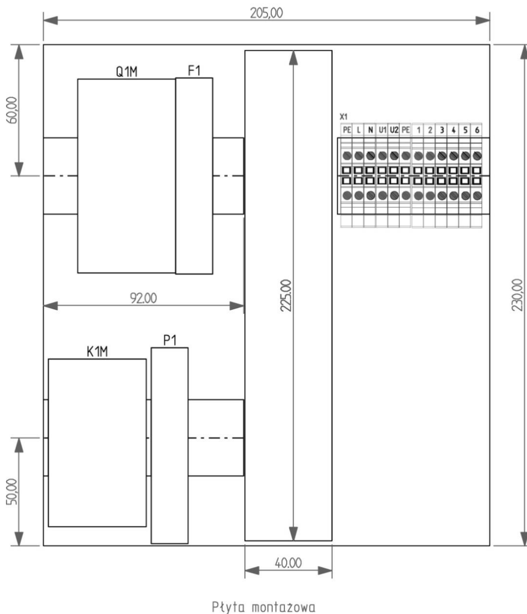
Rys. 6 Płyta montażowa zespołu elektrycznego urządzenia HARD-1000-S
