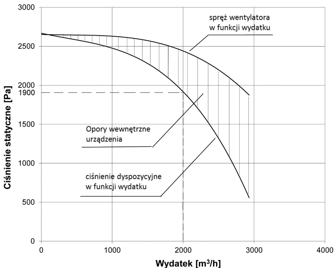
Rys. 1. Charakterystyka przepływowa urządzenia BIG-2000/Ex
