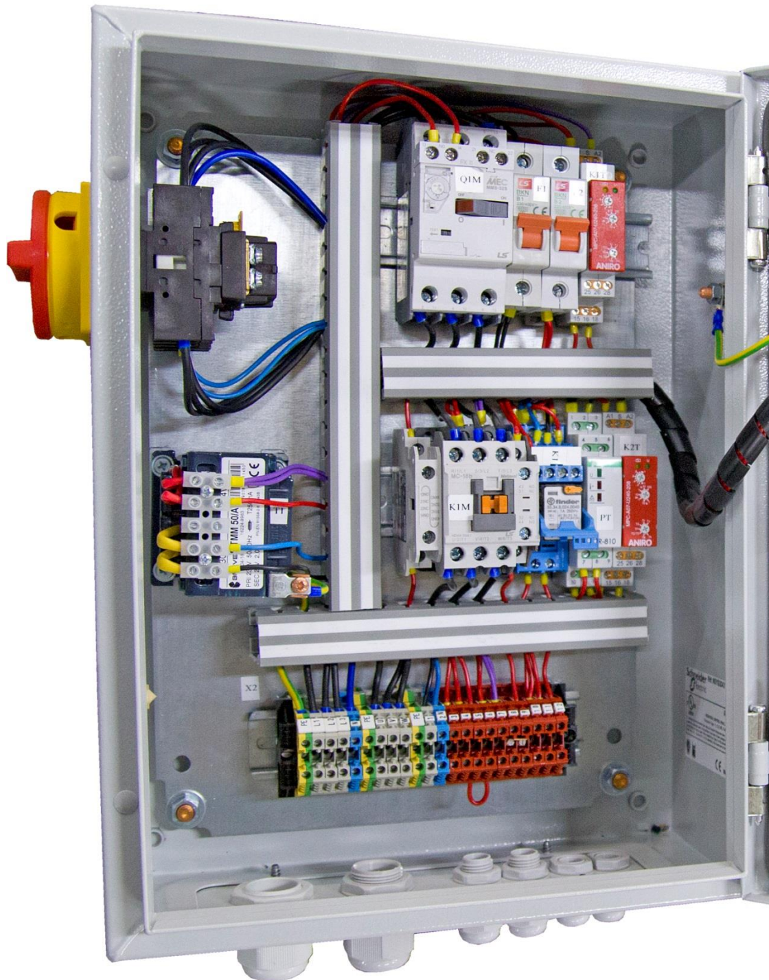
Rys. 10. Rozdzielnica A1, zespół sterujący
