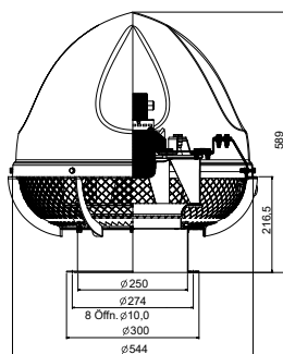
geräuschkämpfender Dachuntersatz TPD-250-N
