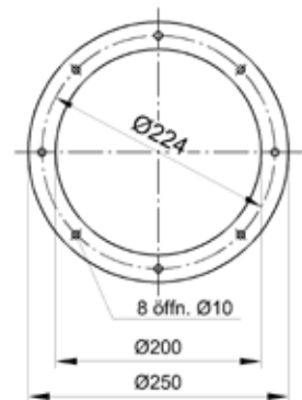
schalldämpfender Dachuntersatz TPDC-200-N
