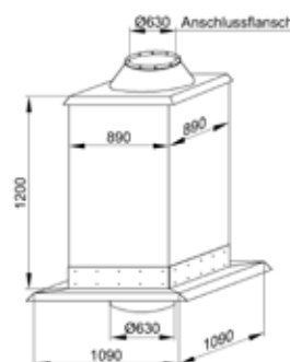
schalldämpfender Dachuntersatz TPDC-630-N
