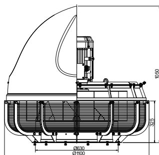
schalldämpfender Dachuntersatz TPD-630-N
