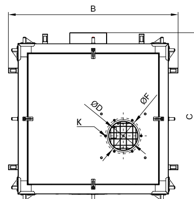
Draufsicht
