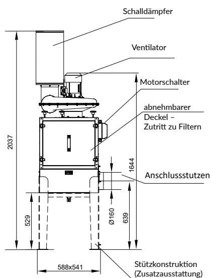
MISTOL-1000
