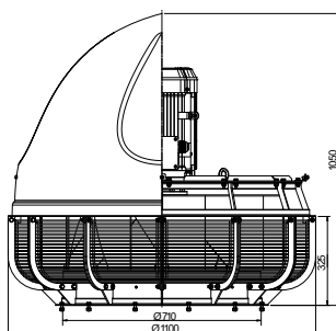
schalldämpfender Dachuntersatz TPD-710-N
