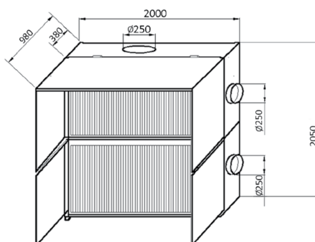
UWT-Werkbank
