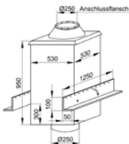
geräuschkämpfender Dachuntersatz TPD-250-N
