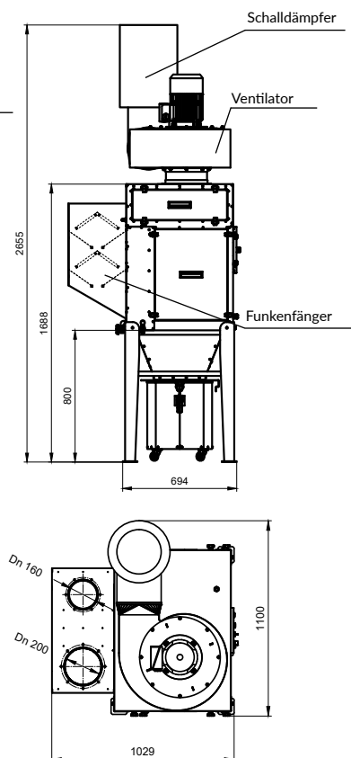
STRONG-2000-N
