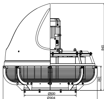
schalldämpfender Dachuntersatz TPD-500-N
