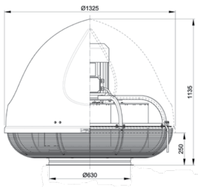
Schalldämpfender Dachuntersatz TPD-630-N
