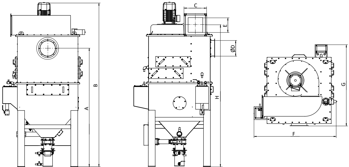
WET-4000-N
