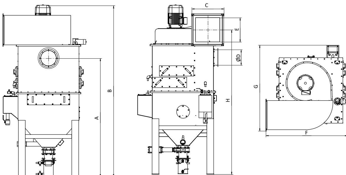
WET-ALU-6000/Ex
