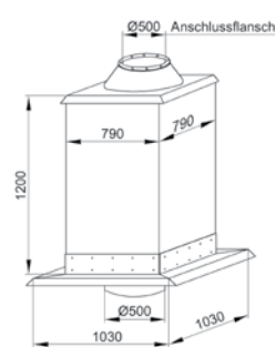
schalldämpfender Dachuntersatz TPDC-500-N
