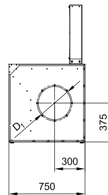
Seitenansicht
