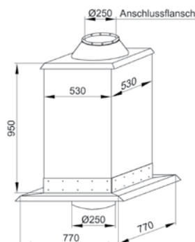
geräuschkämpfender Dachuntersatz TPDC-250-N
