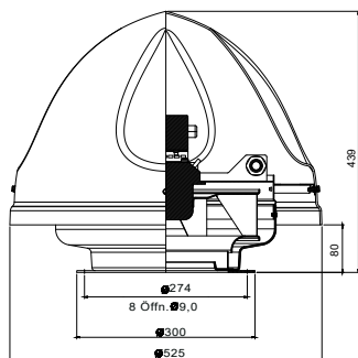
geräuschkämpfender Dachuntersatz TPD-250-N
