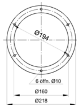
schalldämpfender Dachuntersatz TPDC-160-N
