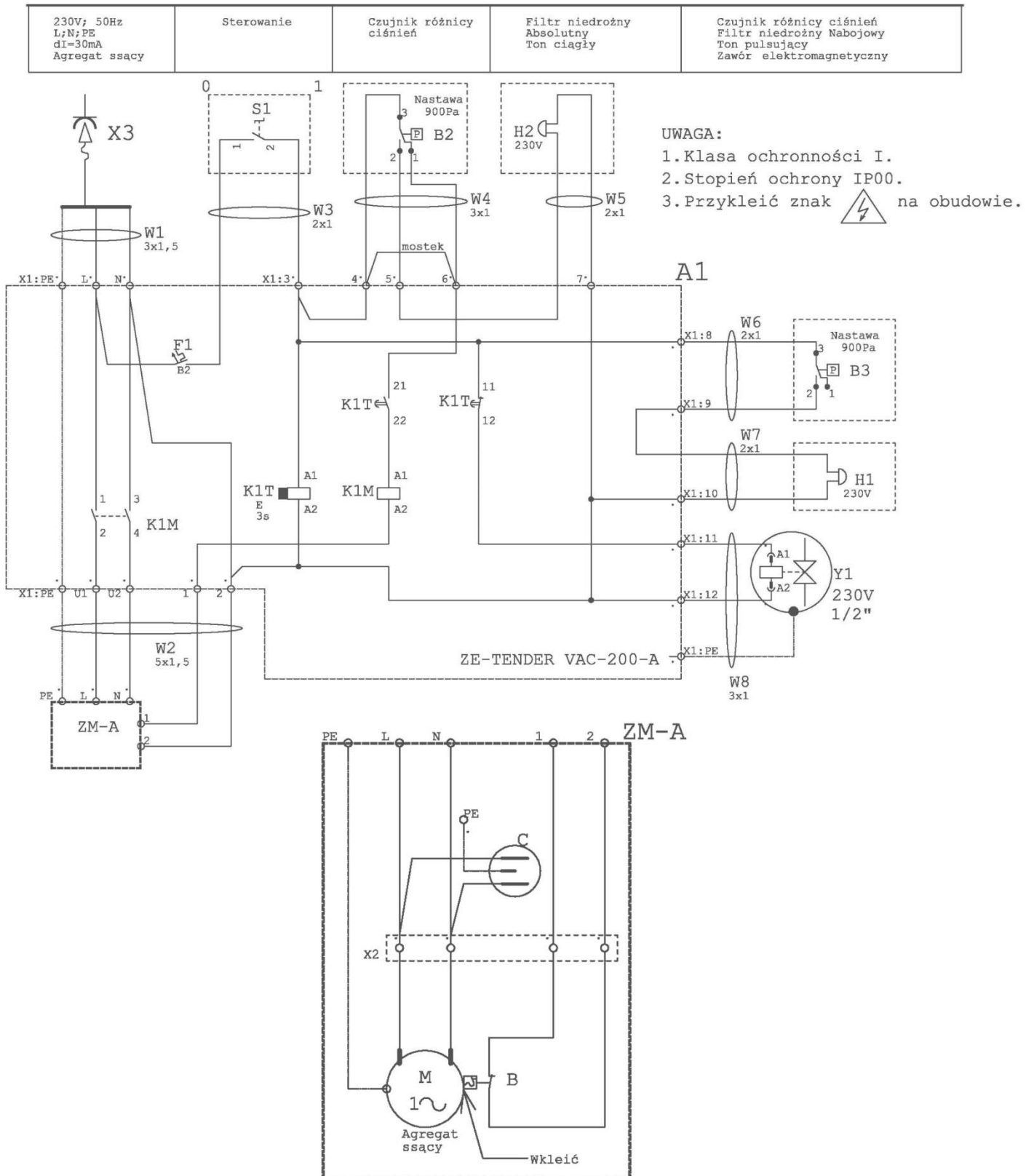
Rys. 4 Schemat elektryczny urządzenia typu TENDER VAC 200-A
