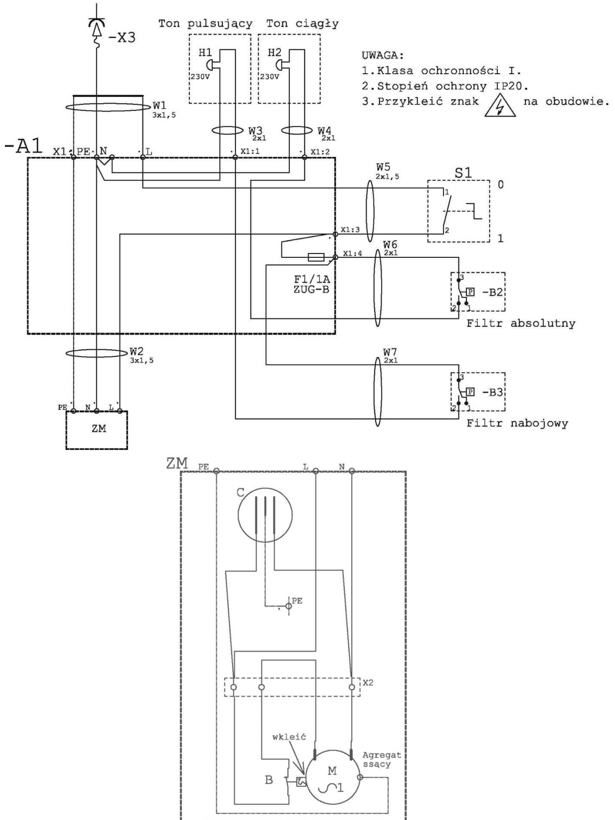
Rys. 3 Schemat elektryczny urządzenia typu TENDER VAC 200-S
