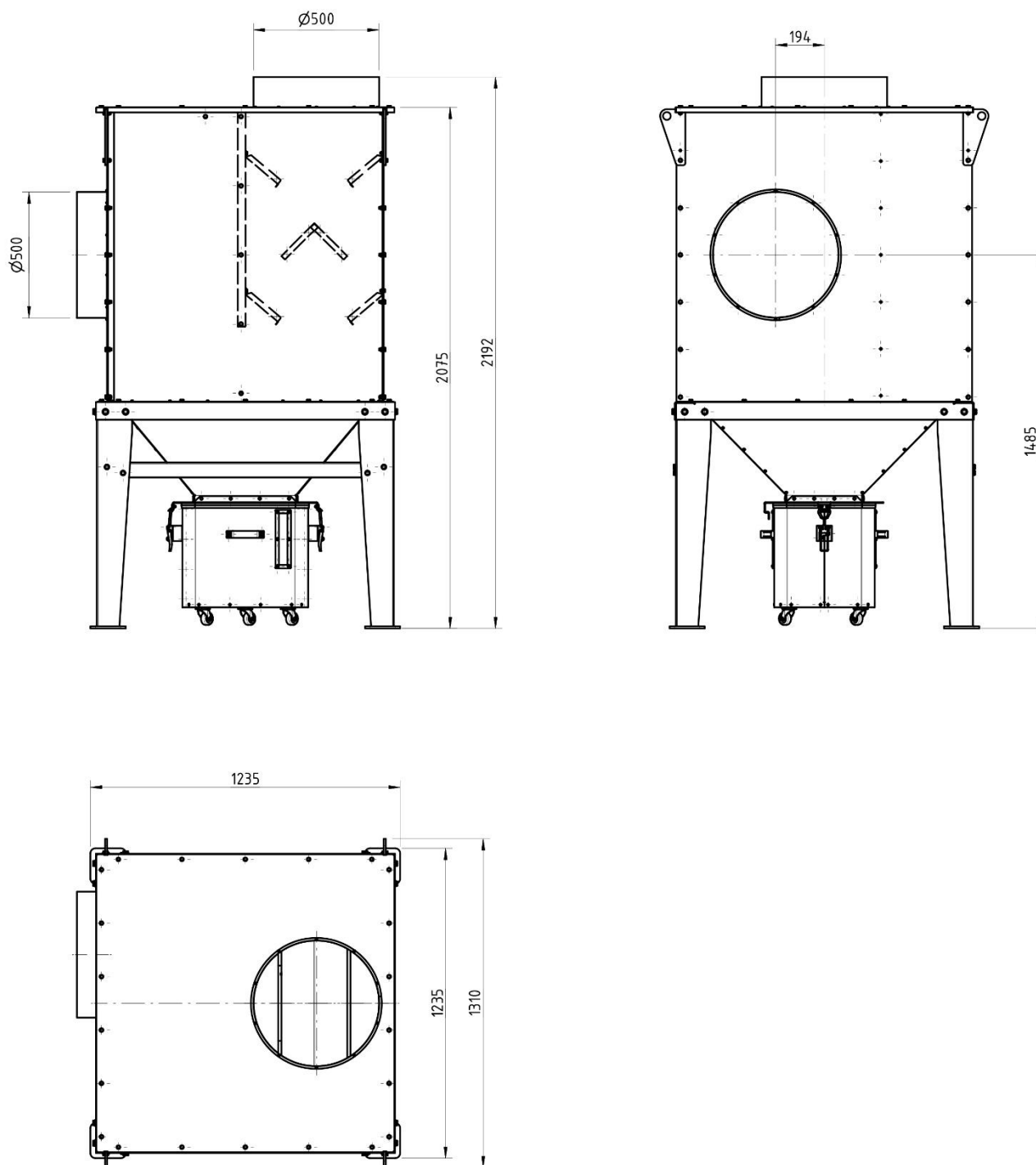
Rys. 1 Budowa i wymiary separatora SEP-UFO-A-10000 – wykonanie lewostronne
