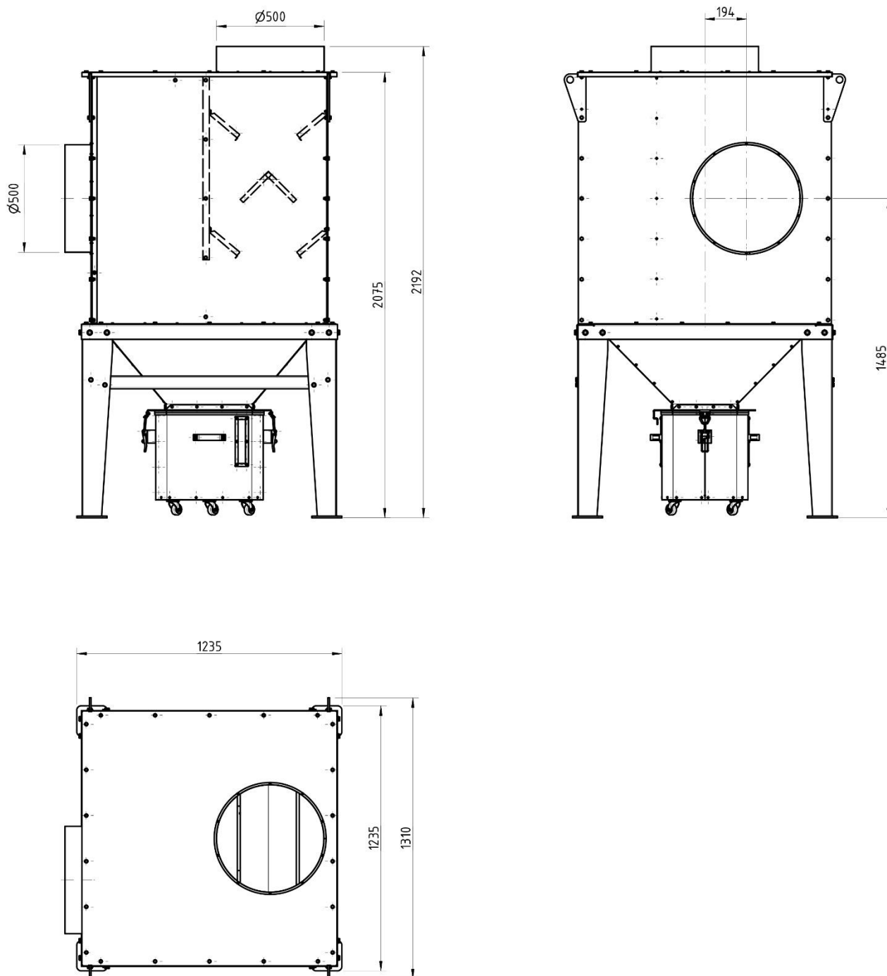
Rys. 2 Budowa i wymiary separatora SEP-UFO-A-10000 – wykonanie prawostronne
