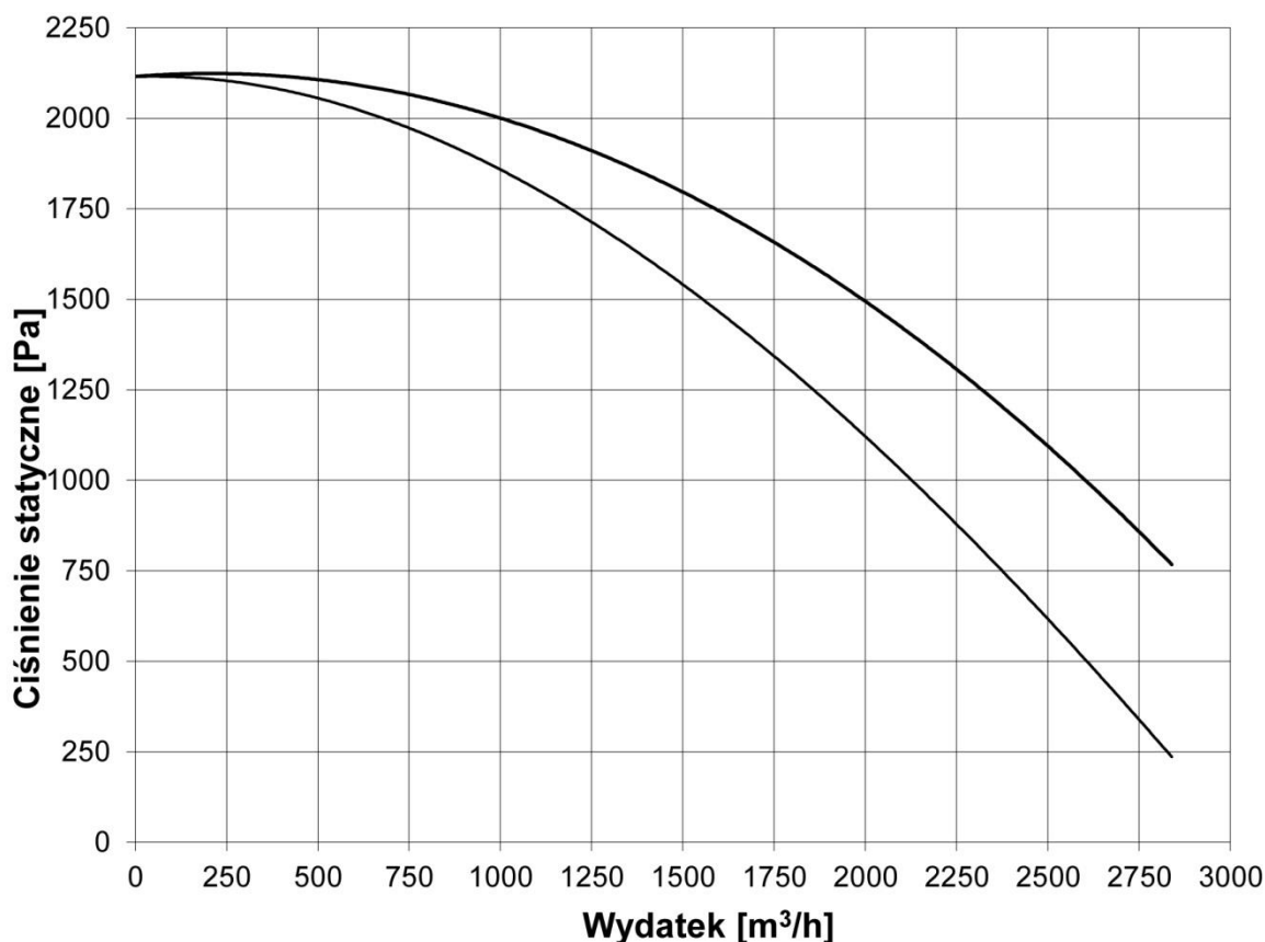
Rys. 1 Charakterystyka przepływowa urządzenia typu MISTOL MIX-2000
