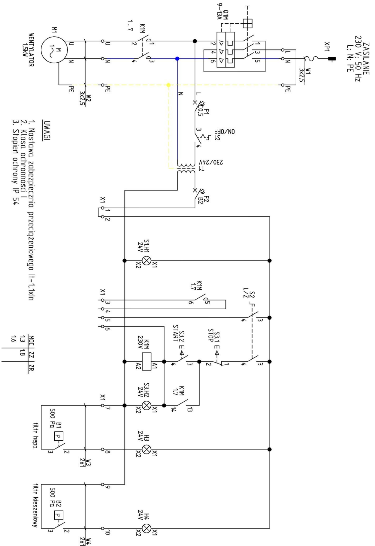
Rys. 3 Schemat elektryczny urządzenia typu MISTOL MIX-2000
