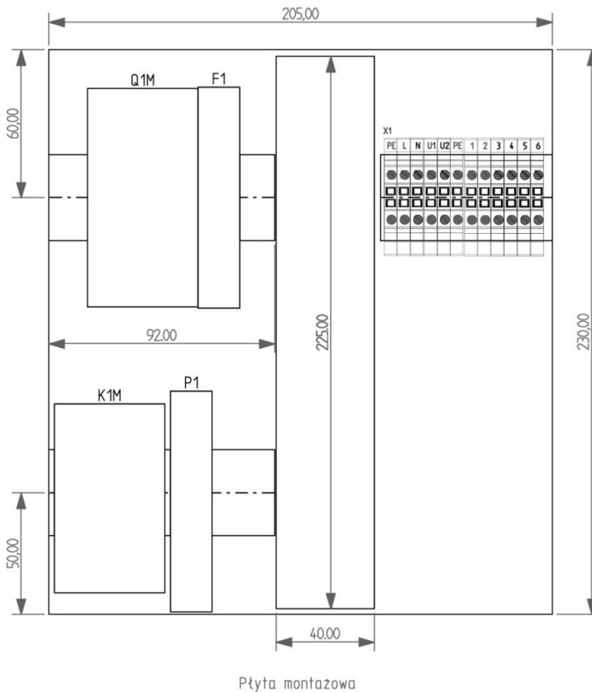
Rys. 7 Płyta montażowa zespołu elektrycznego urządzenia HARD-1000-S
