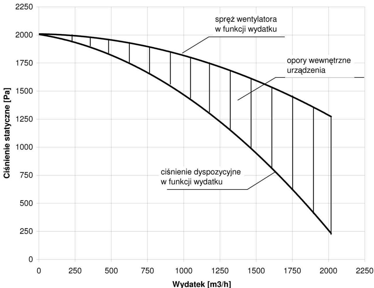
Rys 1 Charakterystyka przepływowa urządzenia typu HARD-2000-S
