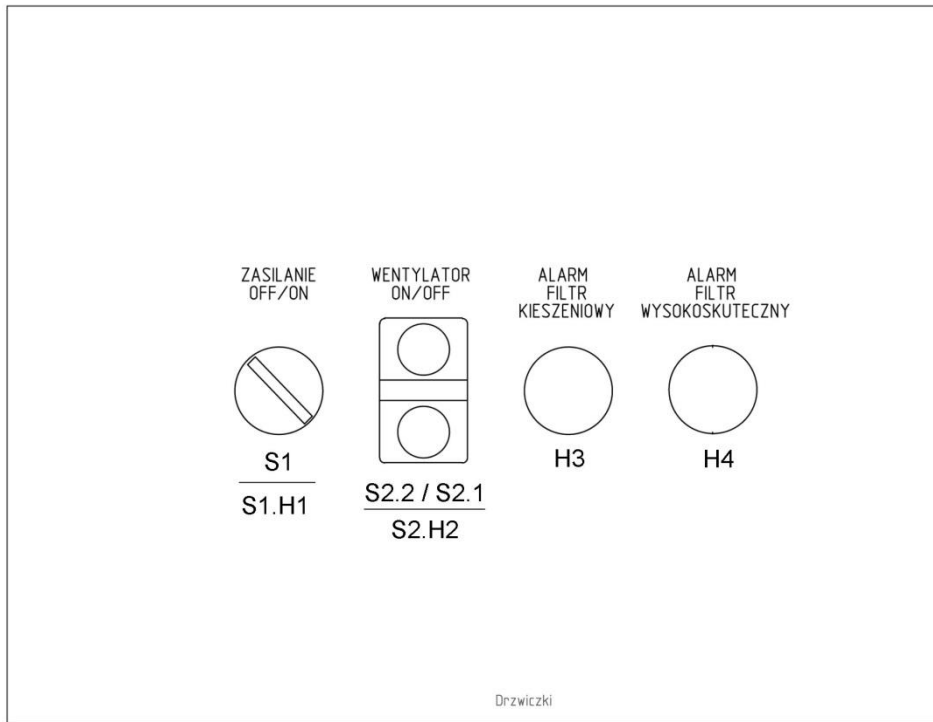
Rys. 6 Zespół elektryczny urządzenia typu HARD-2000-S
