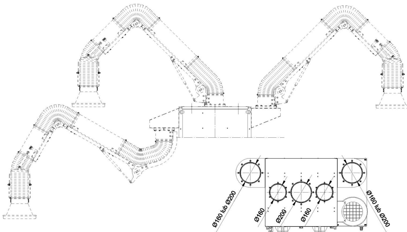
Rys. 4 Sposoby mocowania ramion ERGO LUX
