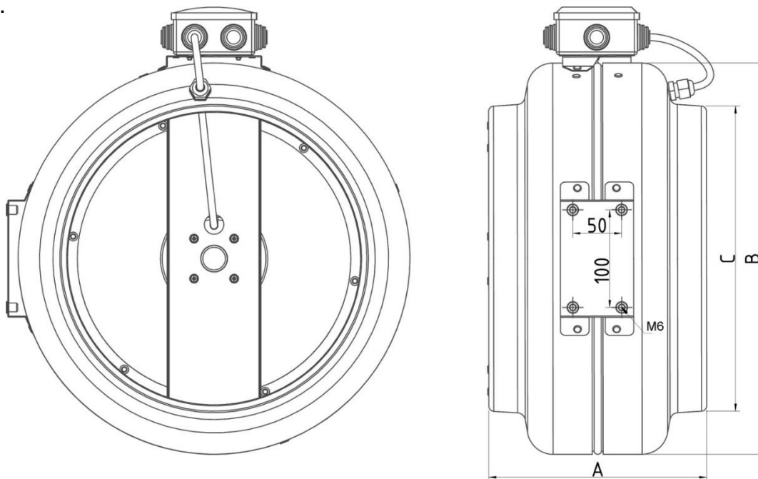
Rys. 1 Wentylator WP-N- budowa i wymiary
