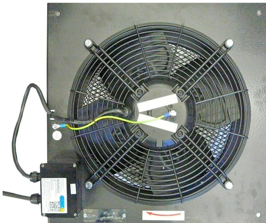
Rys. 3 Rozmieszczenie przewodu uziemiającego i zasilania silnika wentylatora WOK/Ex
