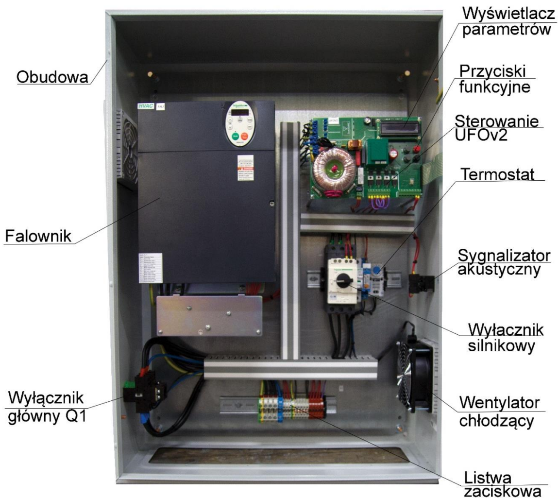
Rys. 7 Rozdzielnica elektryczna ZE-UFO-A – zespoły
