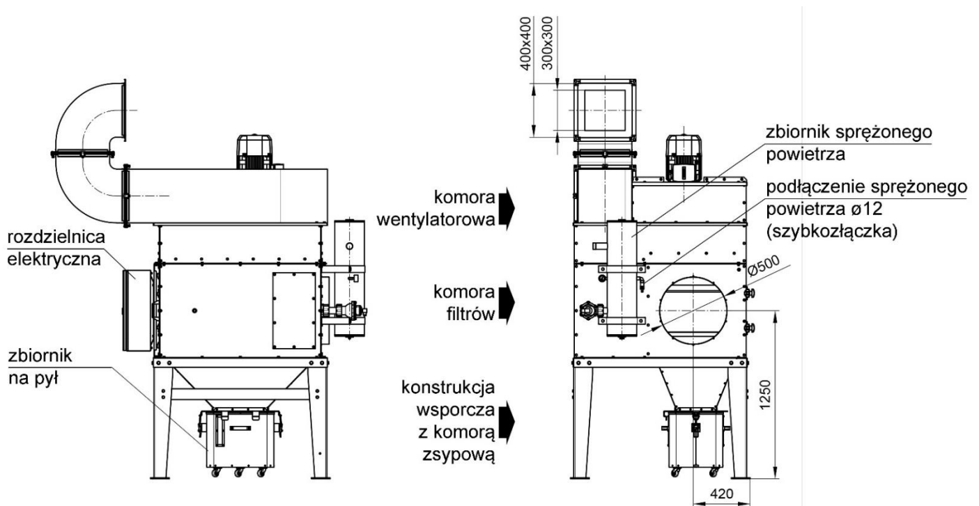
Rys. 3 UFO-A-5000/R RH i LH, budowa i wymiary.
