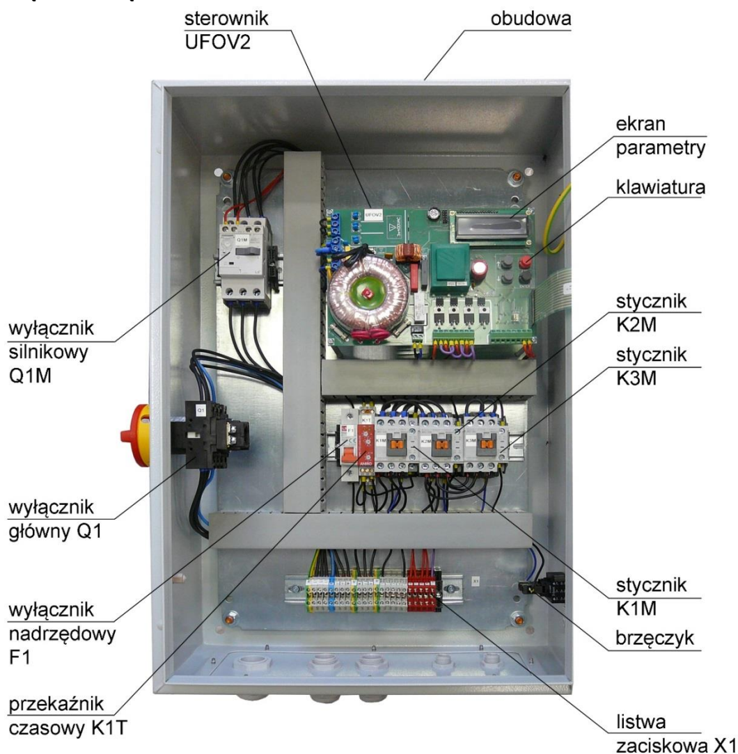
Rys. 7 Rozdzielnica elektryczna ZE-UFO-A – zespoły
