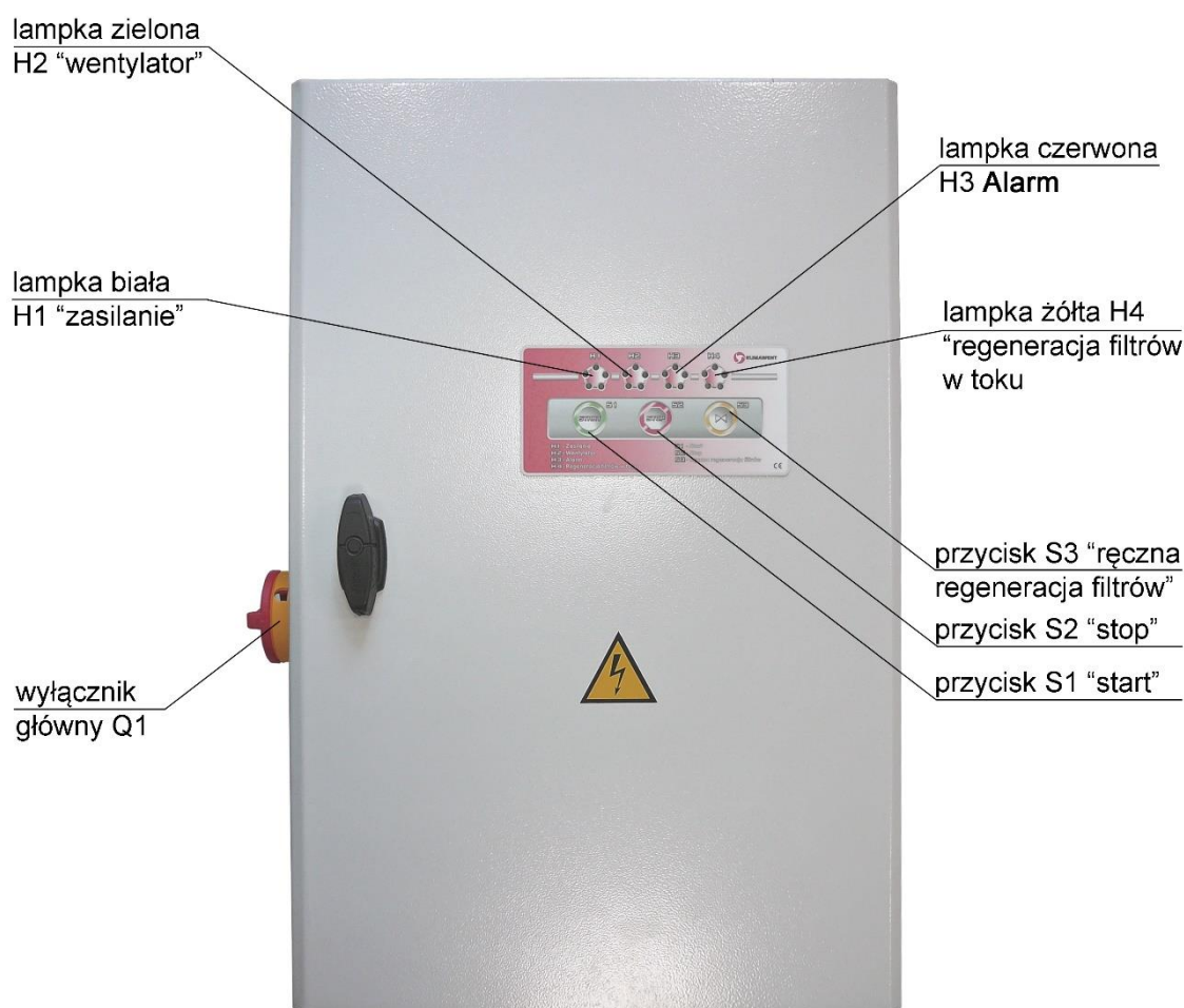
Rys. 5 Rozdzielnica elektryczna – pokrywa
