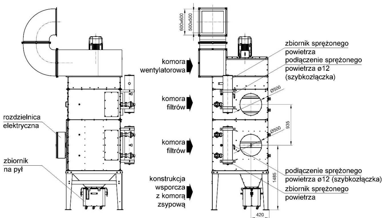
Rys. 3 UFO-A-15000/R, budowa i wymiary
