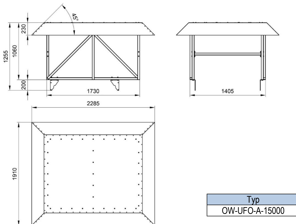
Rys.1 Element dodatkowy – osłona wentylatora instalowana na urządzeniu
