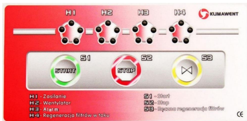
Rys.6 Panel sterowniczy
