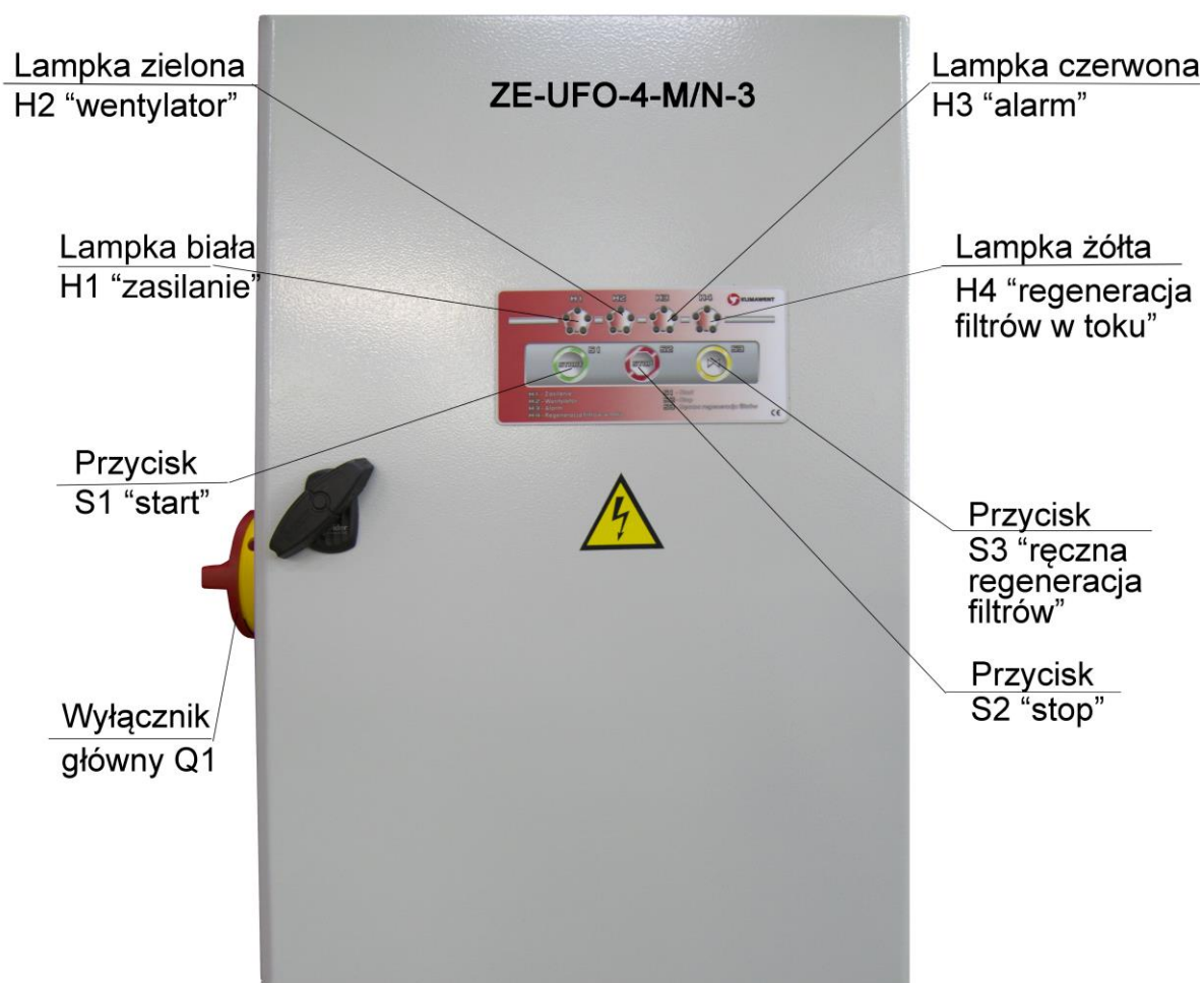
Rys. 5 Zespół elektryczny ZE-UFO-4-M/N-3, elewacja
