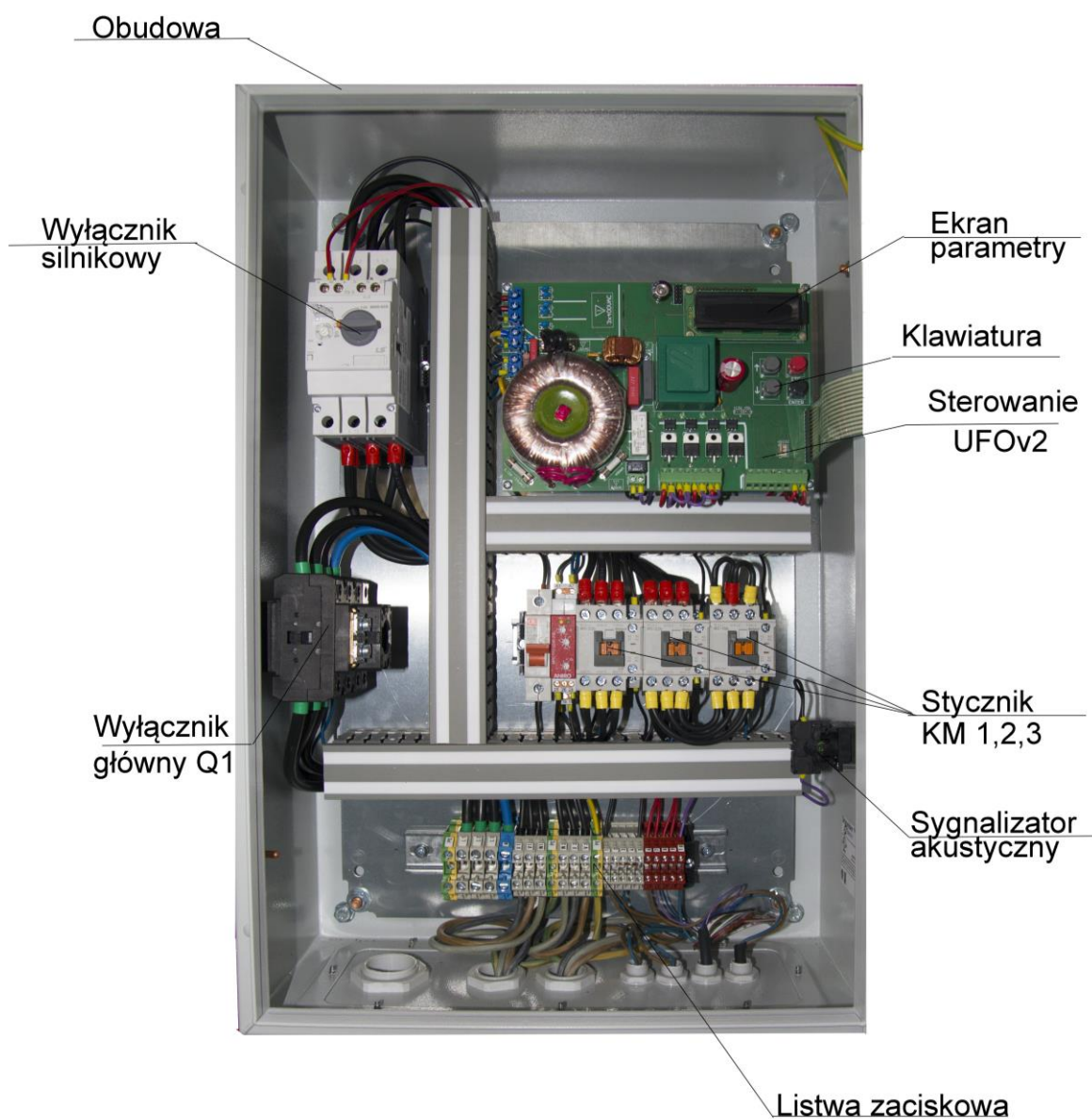
Rys. 7 Zespół elektryczny ZE-UFO-4-M/N-3, wewnątrz
