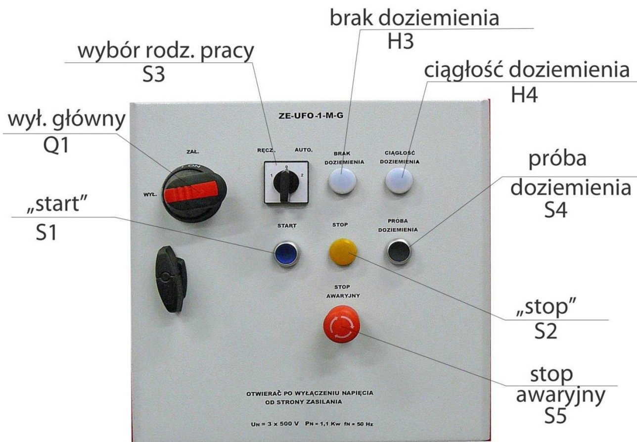
Rys. 2a Zespół elektryczny - drzwiczki
