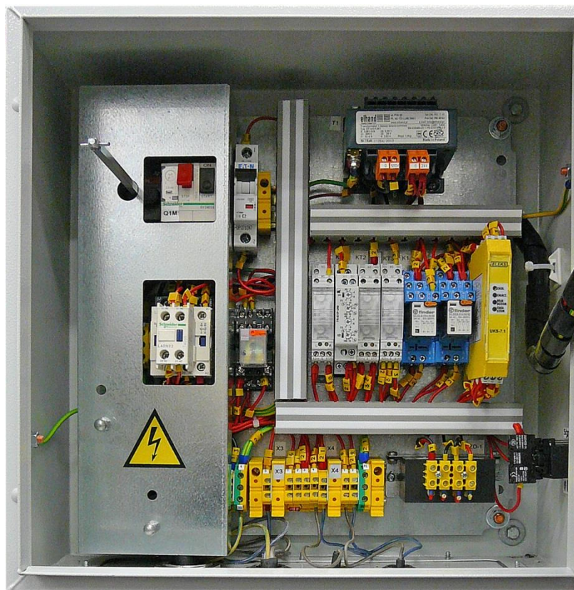
Rys. 2b Zespól elektryczny – wewnątrz skrzynki
