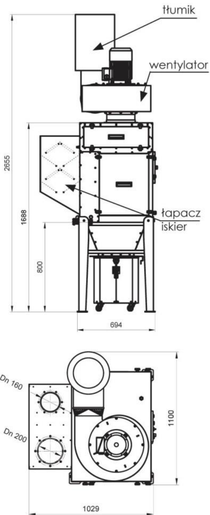
Rys. 2 Budowa i wymiary STRONG-2000-N
