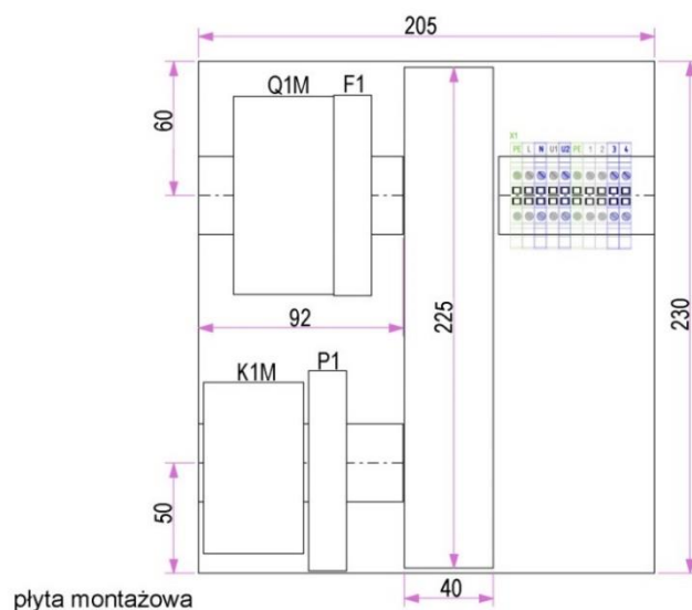
Rys. 5 Zespół elektryczny urządzenia SMOG Filter
