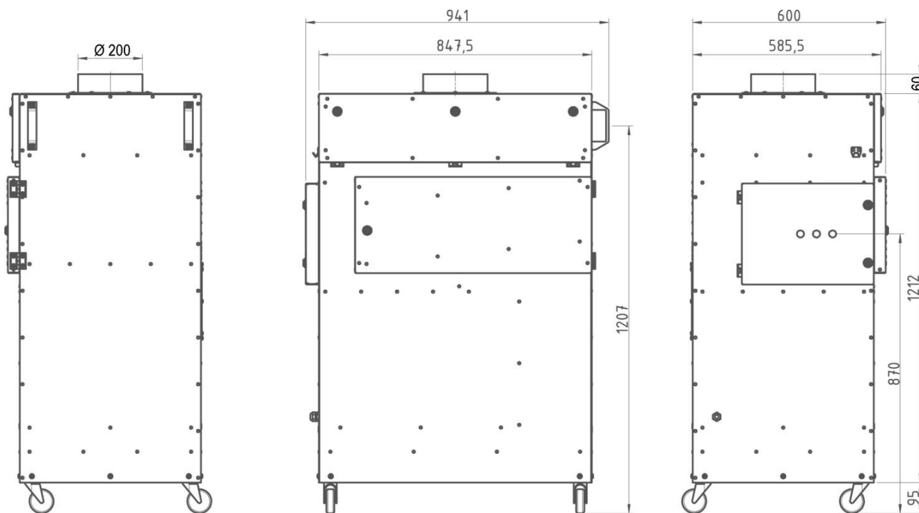
Rys. 2 Wymiary pochłaniacza typu SMOG Filter-400
