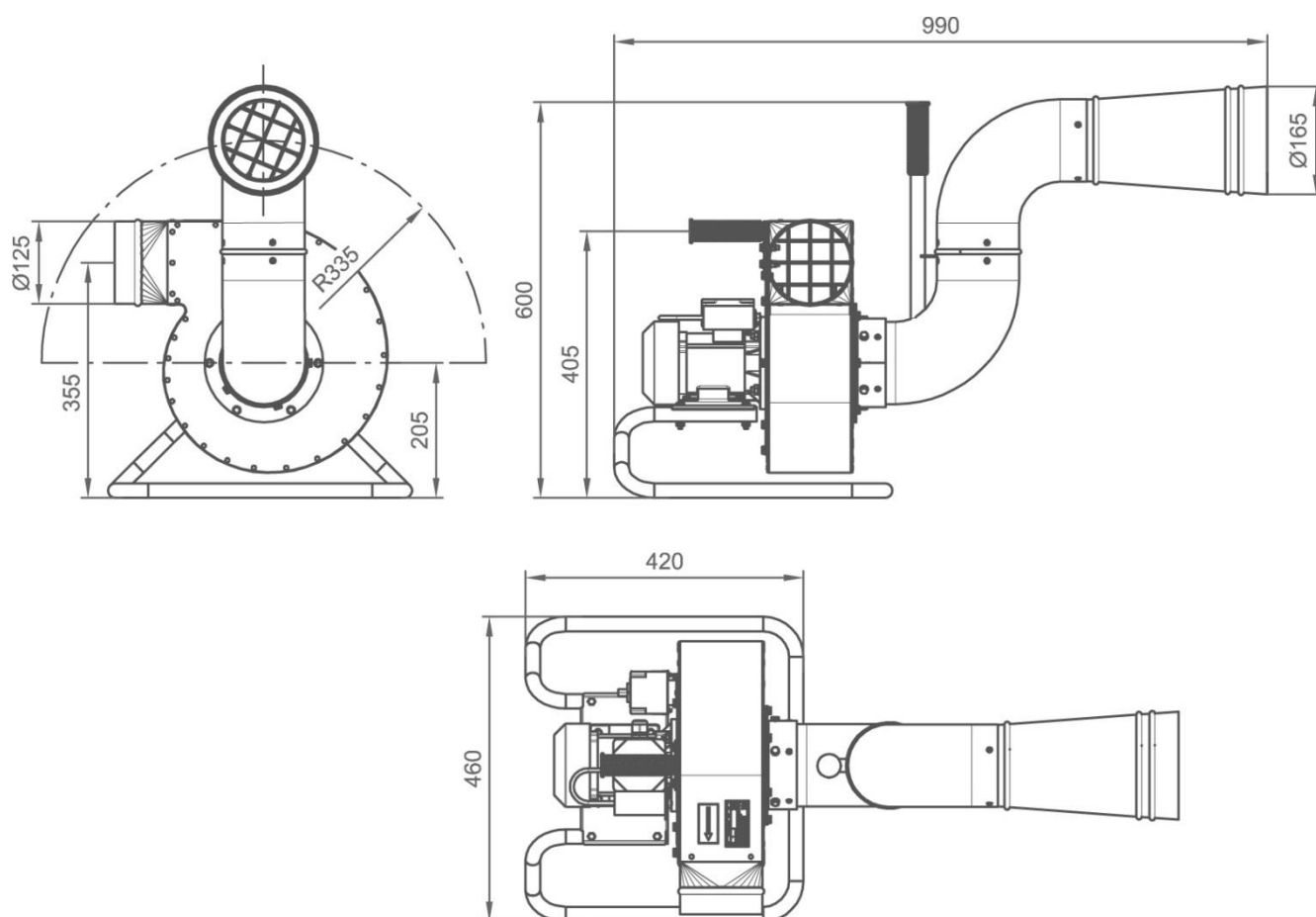
Rys. 1 Odsysacz GEPARD-1000, budowa i wymiary
