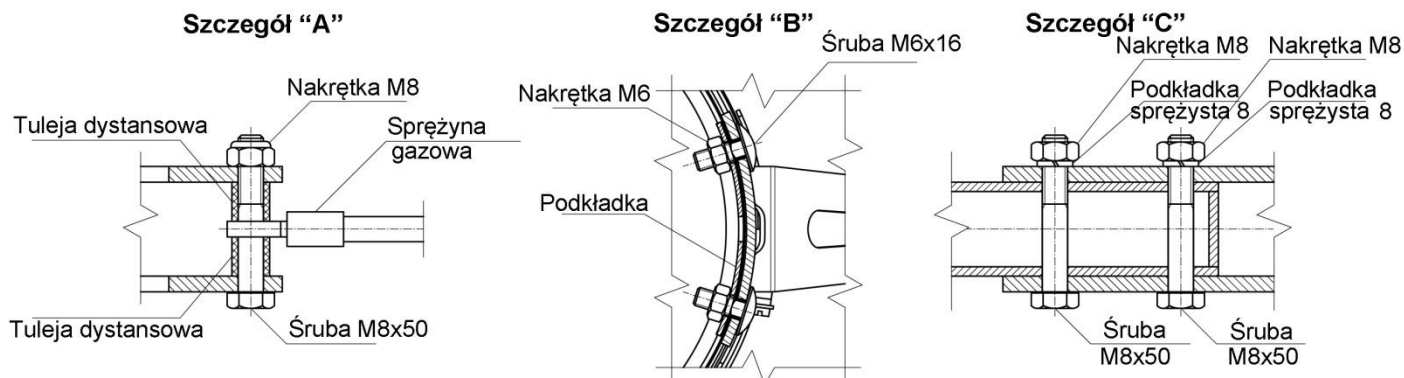
Rys. 5 Montaż ramion ssących wiszących typu ERGO LUX
