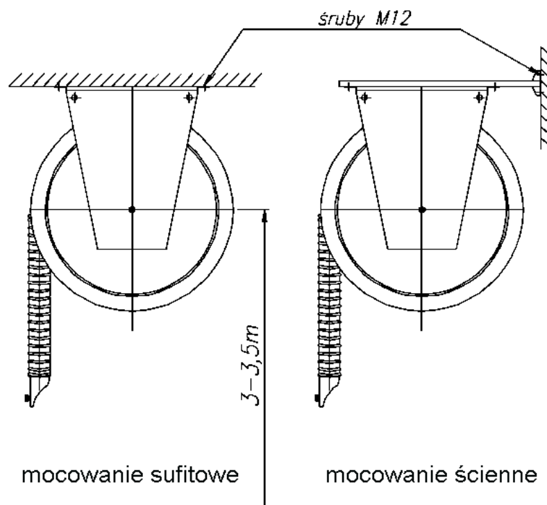
Rys. 8 Montaż odsysacza na stanowisku
