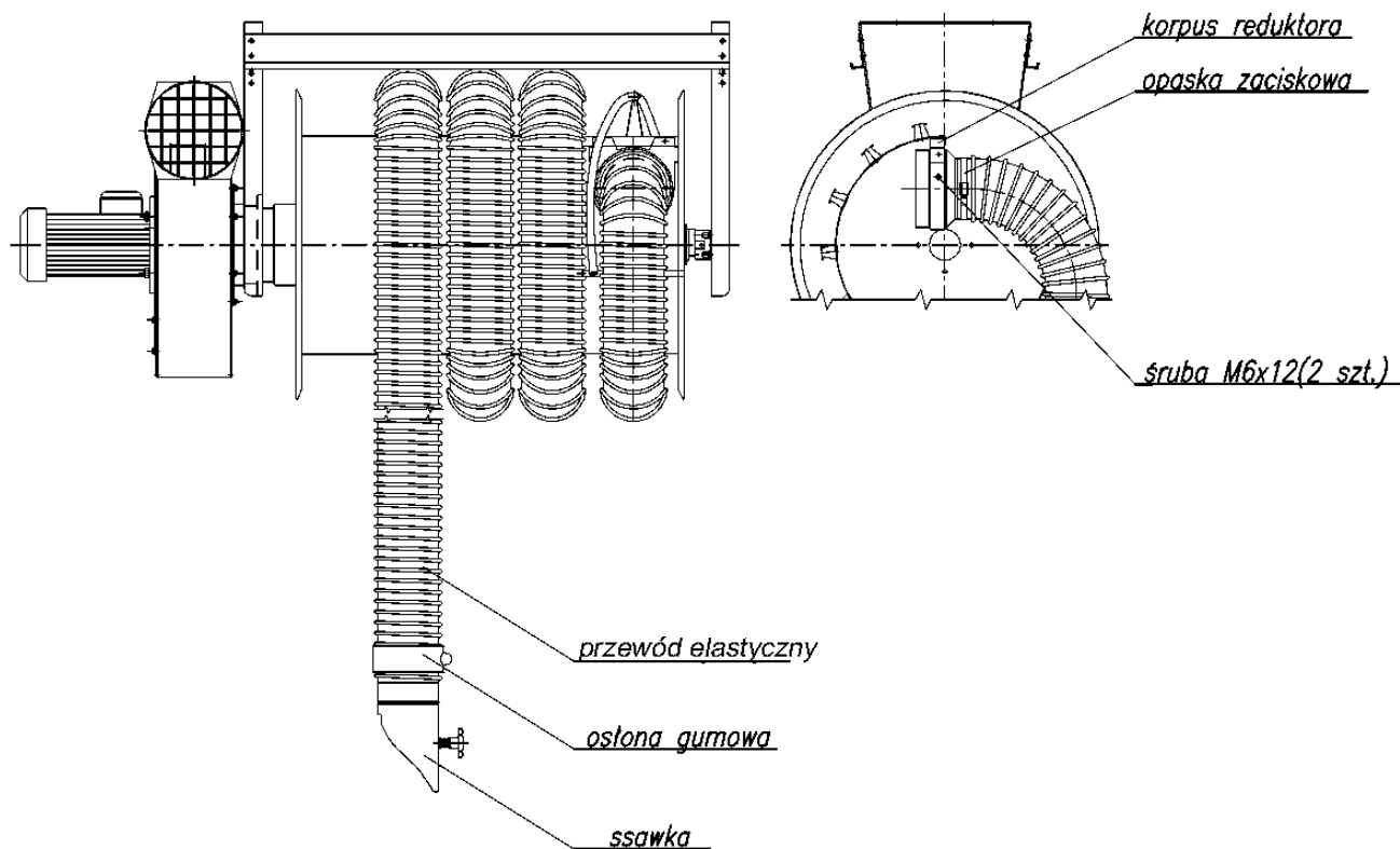
Rys. 3 Mocowanie zestawu węzowego
